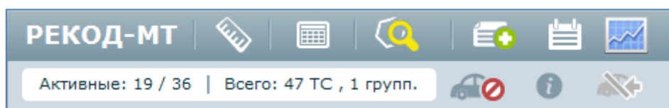
Рисунок 5 - Панель инструментов
