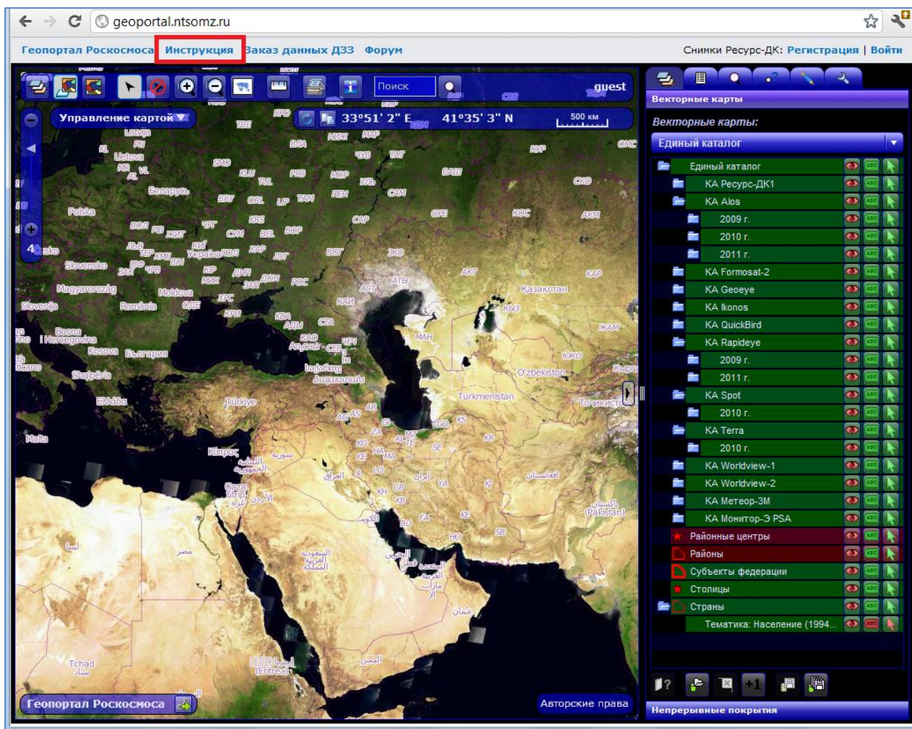
Рисунок 21 – Геопортал Роскосмоса
