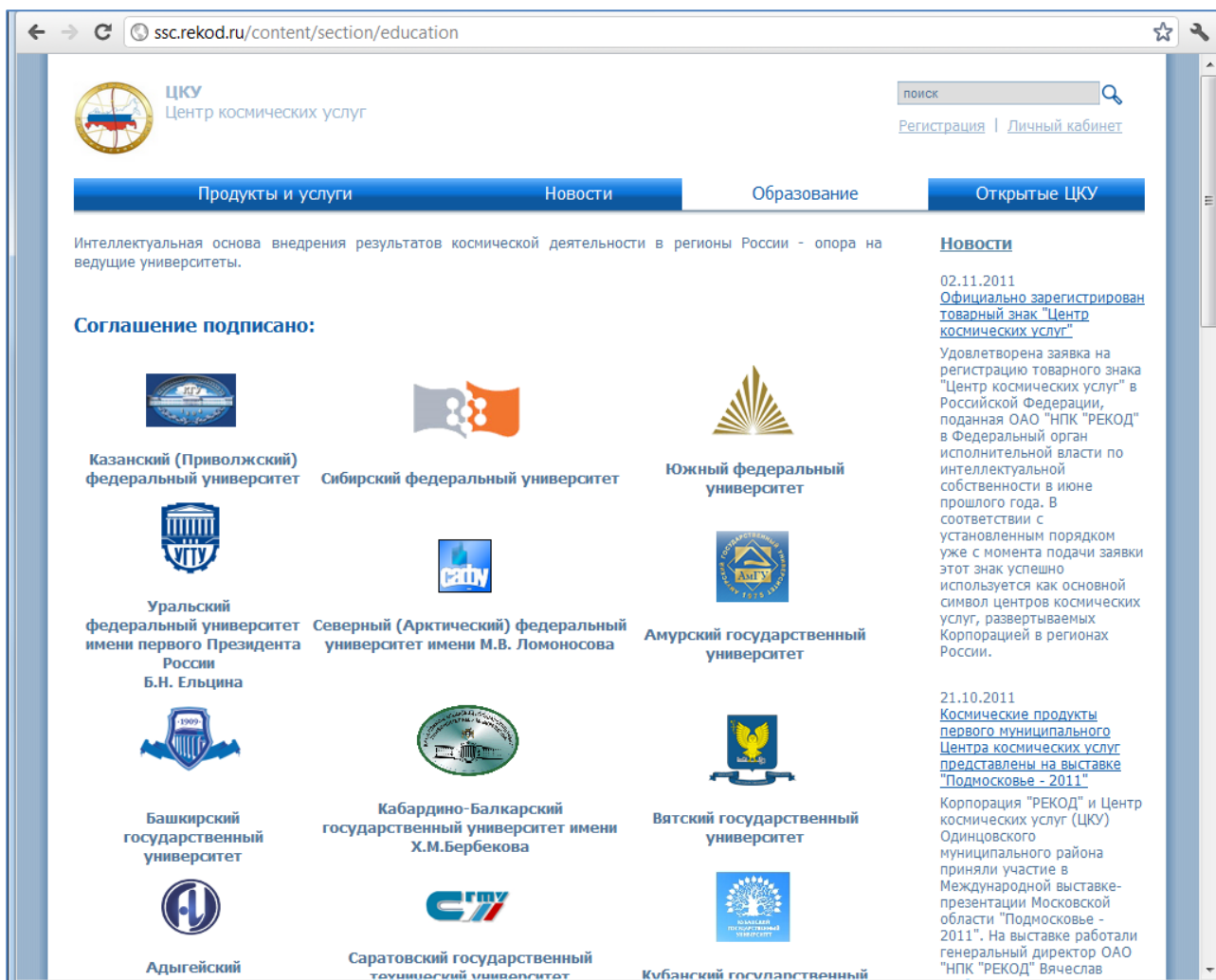
Рисунок 16 – Блок «Образование»
