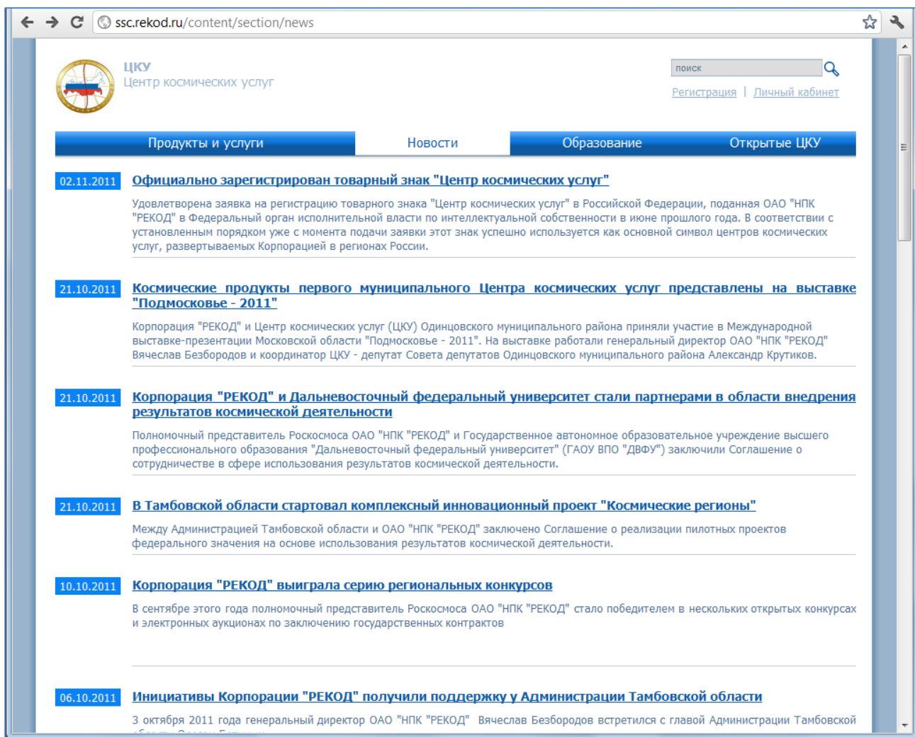
Рисунок 14 – Блок «Новости»
