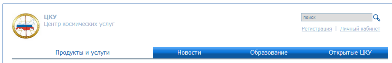
Рисунок 8 – Меню Программы
